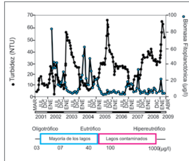
Fig. 5.9. Variación temporal de la turbidez y biomasa fitoplanctónica en Laguna del Sauce. La información presentada corresponde a los promedios mensuales del registro diario de la fuente de agua por parte de la OSE-UGD. La localización de esta estación de muestreo puede ser consultado en el Anexo 1. La escala inferior indica la correspondencia entre la biomasa fitoplanctónica y el estado trófico.
