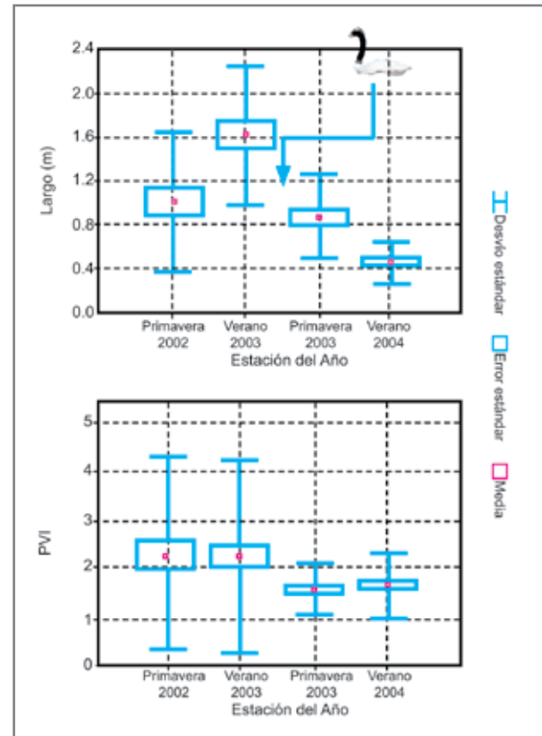
Fig. 5.21. Variación del largo de las plantas y abundancia (PVI) de Egeria densa antes y después de la estancia del Cisne de Cuello Negro durante medio año. Los valores indican la media, error estándar y desvío estándar de casi 100 puntos de muestreo localizado en Laguna del Potrero. Es interesante destacar la disminución de los valores medios y la reducción en la variabilidad de los dos atributos analizados de la población de Egeria densa . El Cisne remueve las hojas de las secciones superficiales, en algunos casos el tallo se corta generando considerables bancos de tallos (de 10 a 40 cm) sin hojas en los márgenes.
