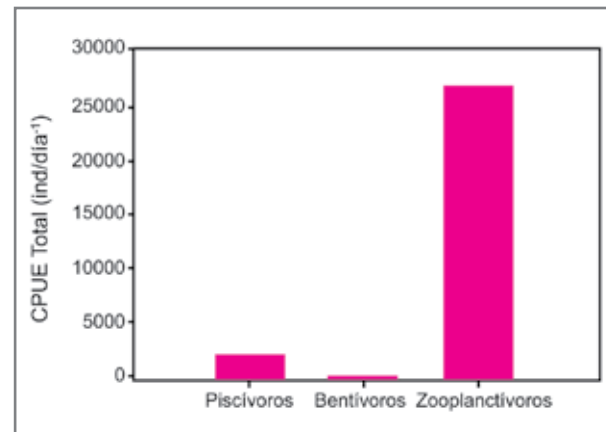
Fig. 5.15. Captura de peces expresada en base diaria (24 horas). La clasificación trófica enfatizó la potencialidad de incluir peces o zooplancton en la dieta. Se incluyen también los peces que se alimentan en el fondo (bentívoros). La información comprende las capturas de Laguna del Sauce, Cisne y Potrero.
