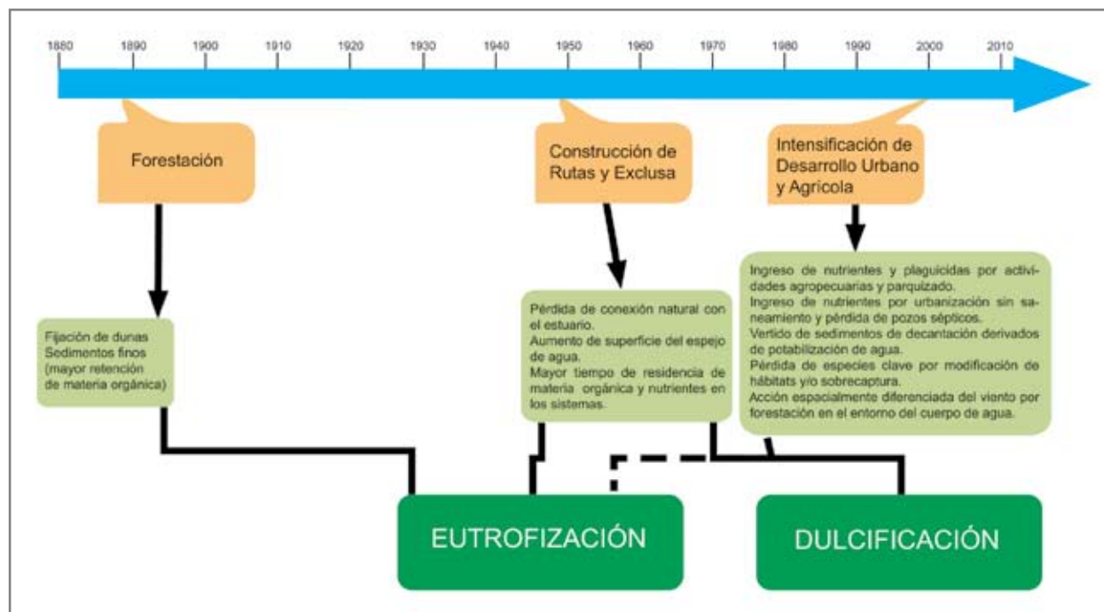
Fig. 5.8.- Principales actividades humanas desarrolladas en sistemas acuáticos del sudeste del Uruguay y su relación con los principales procesos inferidos para los mismos. Fuente: Inda, 2009.
