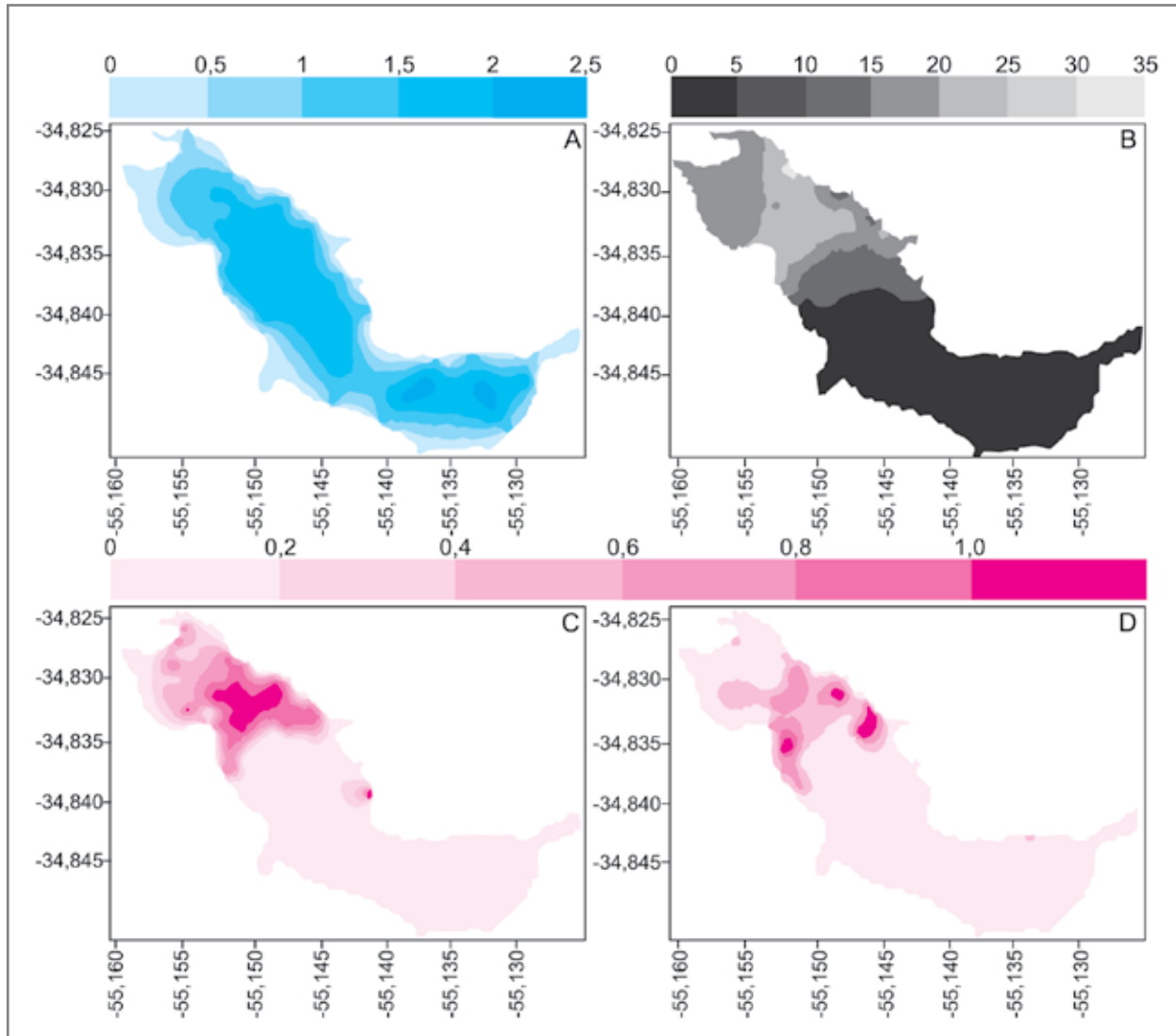
Fig. 5.18. A. Mapa batimétrico de Laguna del Potrero, la escala de profundidades indicada con el gradiente de colores corresponde a metros. B. Variación espacial de la transparencia del agua estimada como profundidad del minidisco de Secchi (en cm), mayor profundidad corresponde a mayor transparencia del agua. C y D. Distribución espacial de la abundancia de Egeria densa y Ceratophyllum demersum , respectivamente, en el otoño del 2008. La abundancia se expresa en porcentaje del volumen de la columna de agua ocupado por plantas (PVI), el 1 corresponde a 100% y el 0 a 0%.
