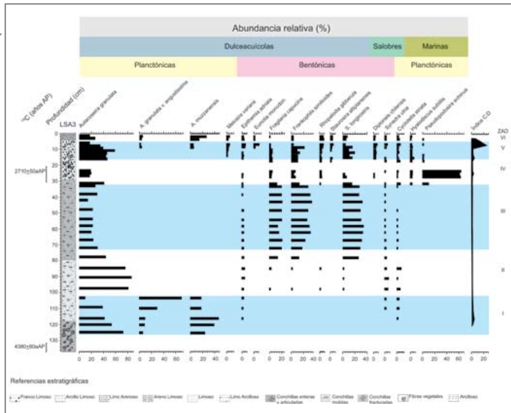
Fig. 5.5. Testigo sedimentario LSA3. Contenido de flora diatomológica e índice C:D (crisofitas versus diatomeas). La parte superior del corer representa los últimos años o décadas y la más profunda el período más antiguo (miles de años). Los proxies utilizados permiten inferir variaciones del estado trófico y de la salinidad del agua (asociado a variaciones pasadas del nivel del mar). Fuente: Inda (2009).
