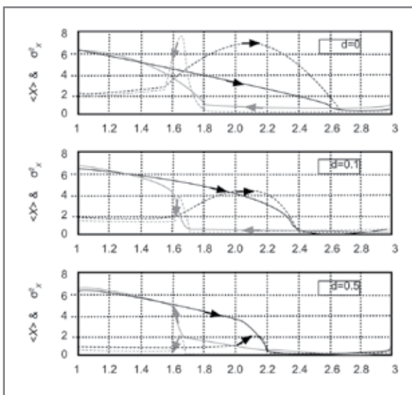
Fig. 11.4. Modelo de pastoreo, abundancia de la vegetación ( X , curvas llenas) y su variancia espacial \sigma_x^2 (líneas de trazos) para K = 7.5 calculado para tasa de consumo c aumentando (negro) y disminuyendo (gris). Resultados para d = 0 (arriba), d = 0.1 (medio) y d = 0.5 .
