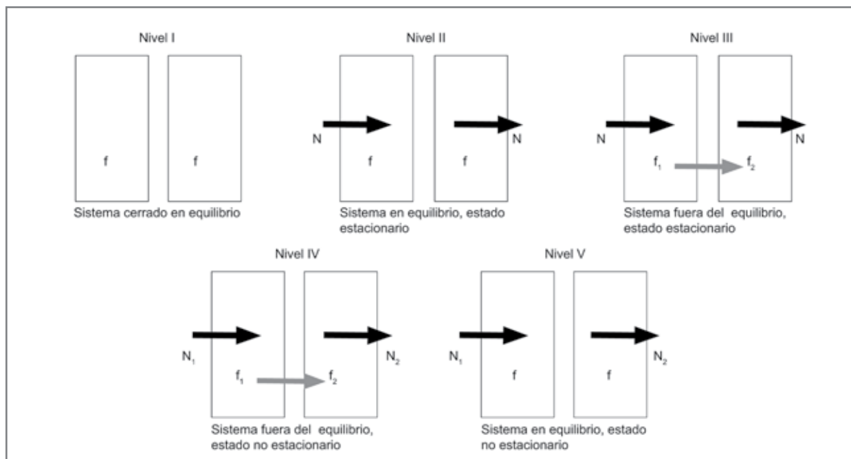
Fig. 10.1. Niveles de complejidad de los modelos de fugacidad (siendo N la tasa de advección y f la constante de fugacidad). Fuente: Wania 2001.
