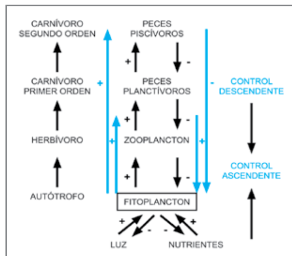
Fig. 4.5. Esquema representativo de las interacciones tróficas directas (por ejemplo herbivoría, depredación, entre otras, se indican en negro) e indirectas (por ejemplo cascada trófica, se indica en azul) que regulan la abundancia y biomasa del fitoplancton. Los signos señalan si los efectos son positivos o negativos. En este esquema se puede comprender por qué un aumento del stock de piscívoros provoca indirectamente un aumento de la presión de herbivoría sobre el fitoplancton.
