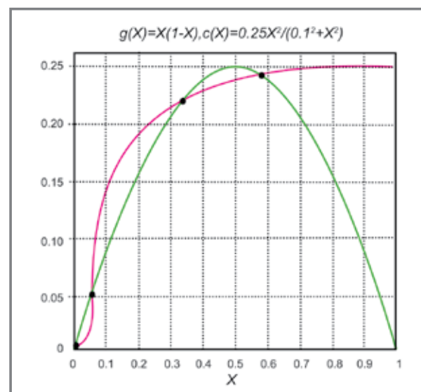
Fig. 11.2. Término de crecimiento logístico (verde) y consumo de Holling tipo III o sigmoideal (curva roja).
