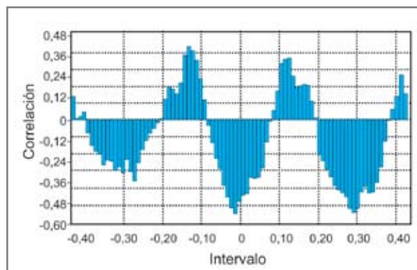
Fig. 5.11. Análisis de correlación cruzada de las series temporales de clorofila y turbidez. El resultado matemático permite establecer la relación inversa entre ambas variables e identificar el periodo de tiempo en que la correlación es positiva. De una forma simple podemos concluir que luego de los incrementos bruscos de turbidez el aumento de la biomasa algal ocurre a partir del año (máximo valor de correlación positiva). El eje de los intervalos indican meses.
